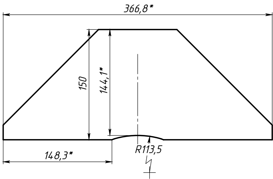
Поз.1 (Корпус) развертка
